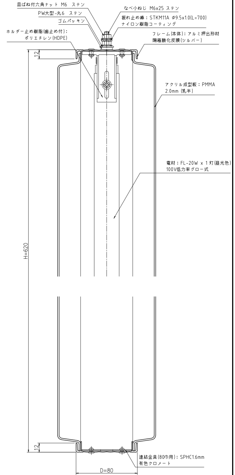
A~A断面詳細図 1:2
