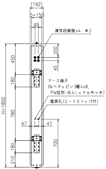
壁面側姿図 1:20
