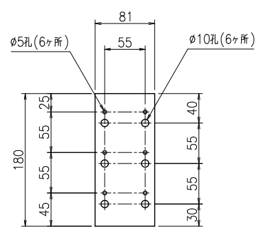
ブラケット部アンカー孔詳細図 1:5
