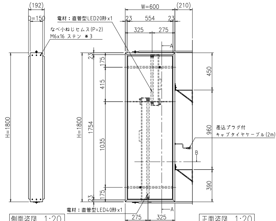
正面姿図 1:20
