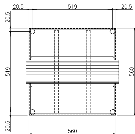
上面姿図(1:10)
