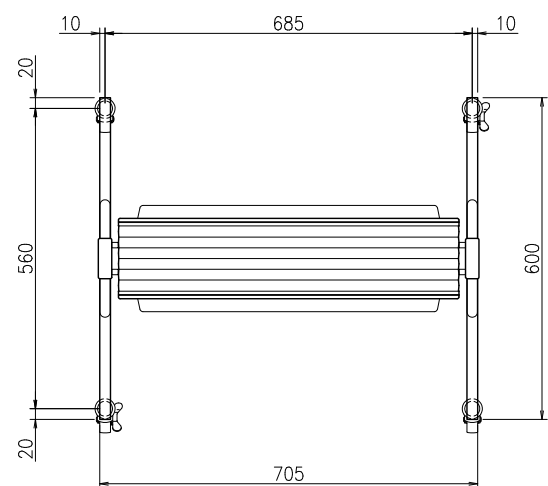
上面姿図(1:10)
