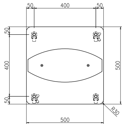
上面姿図(1:10)
