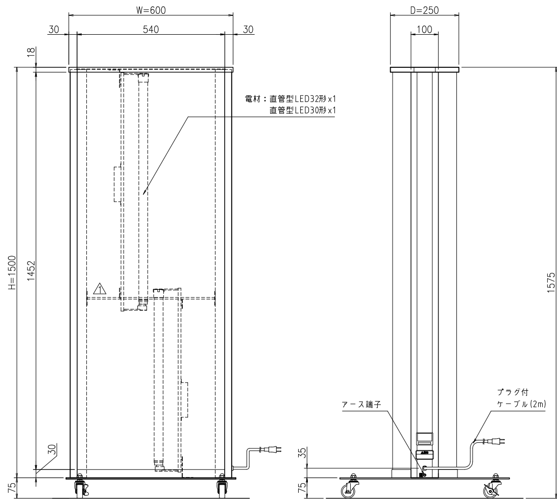
正面姿図(1:10)
