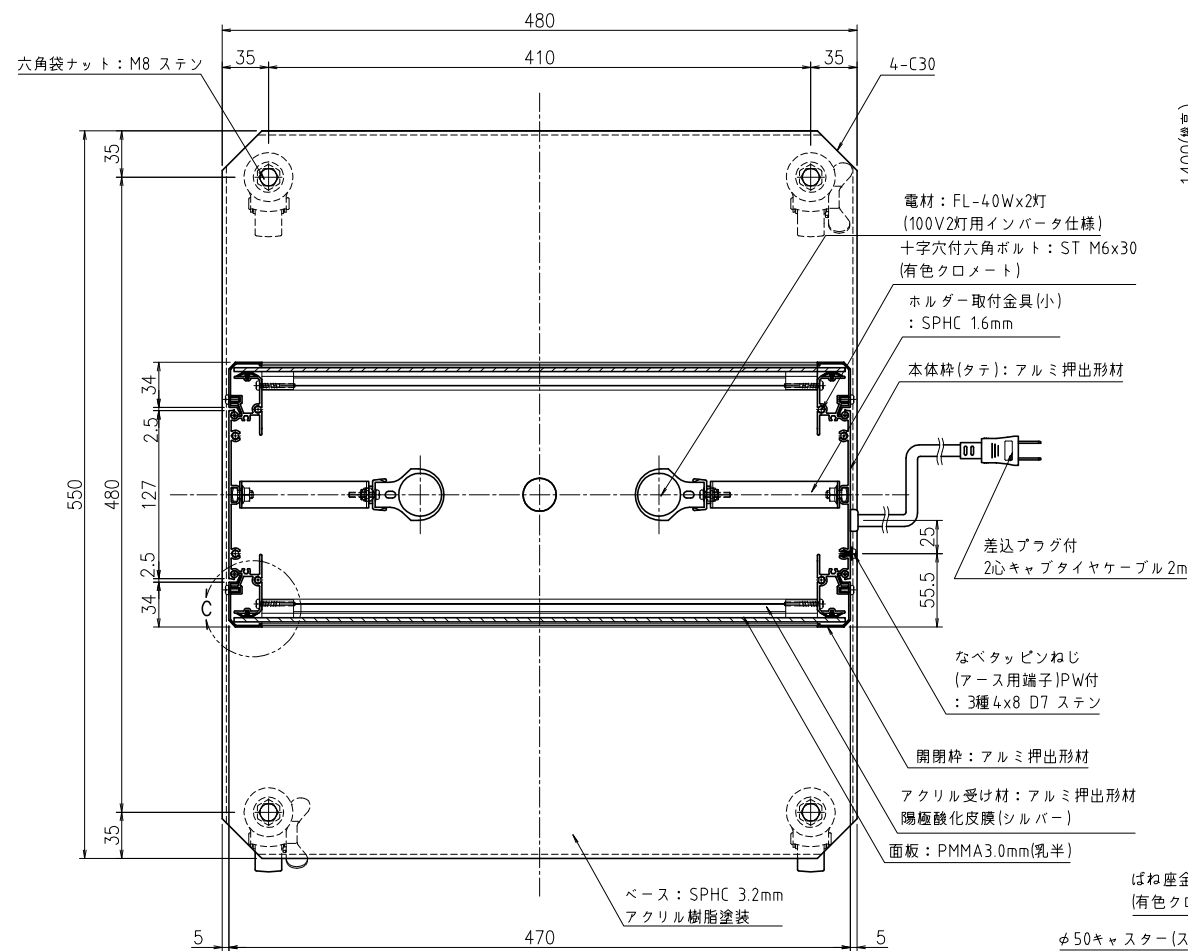
B~B断面詳細図(1:4)
