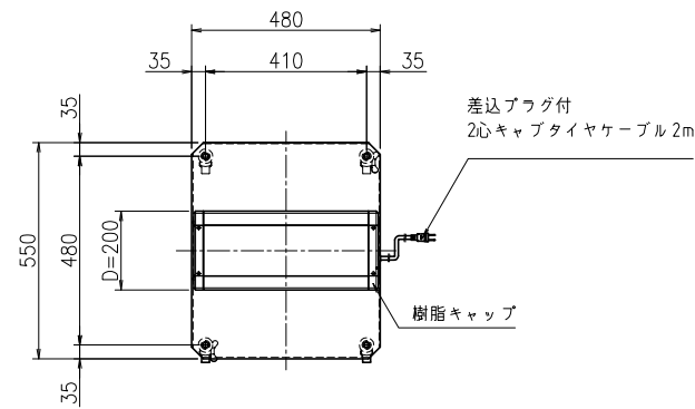
上面姿図(1:15)
