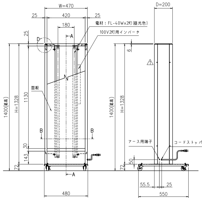
正面姿図(1:15)
