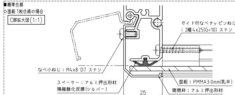
C部拡大図(1:1)
