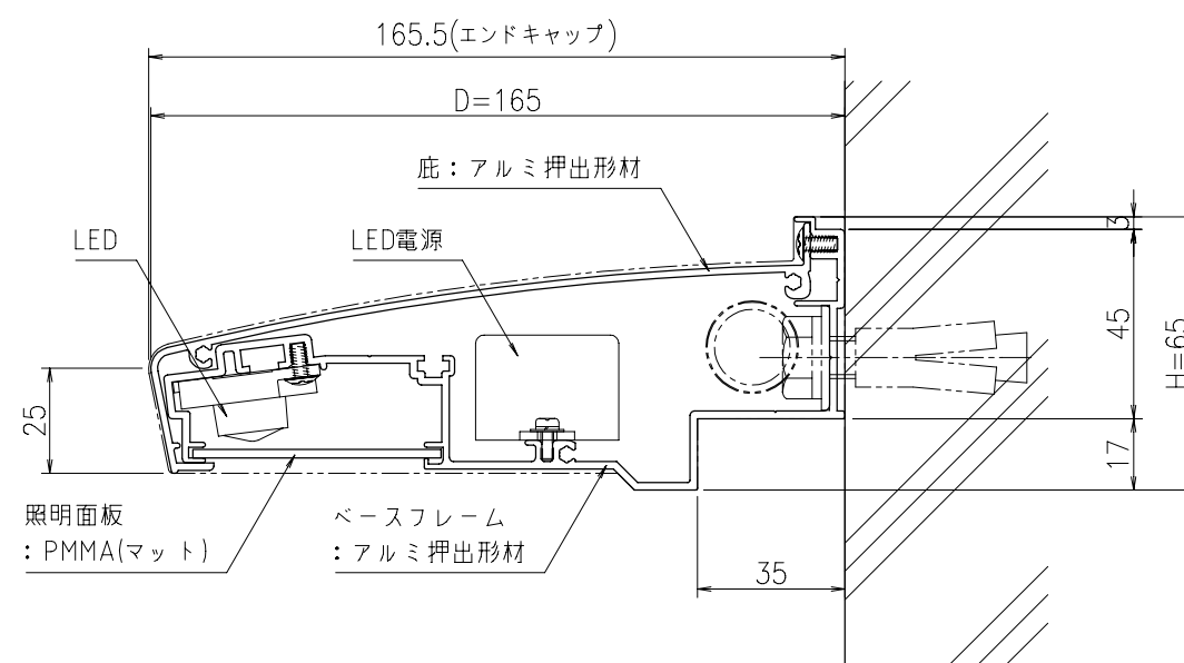
断面詳細図 (1:2)
