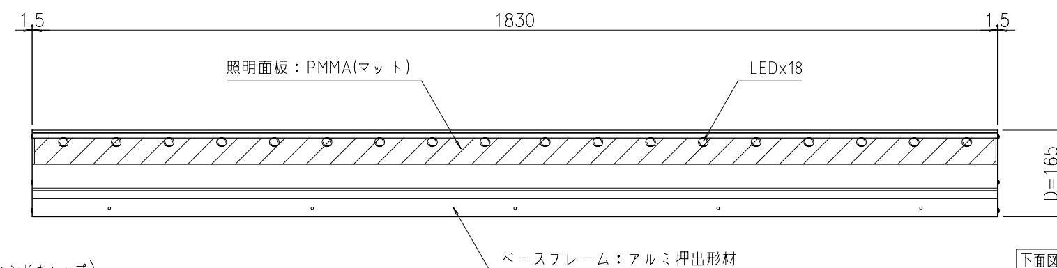
正面図
