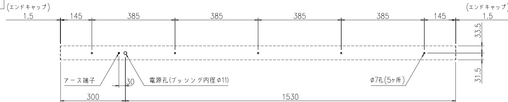
アンカー位置図
