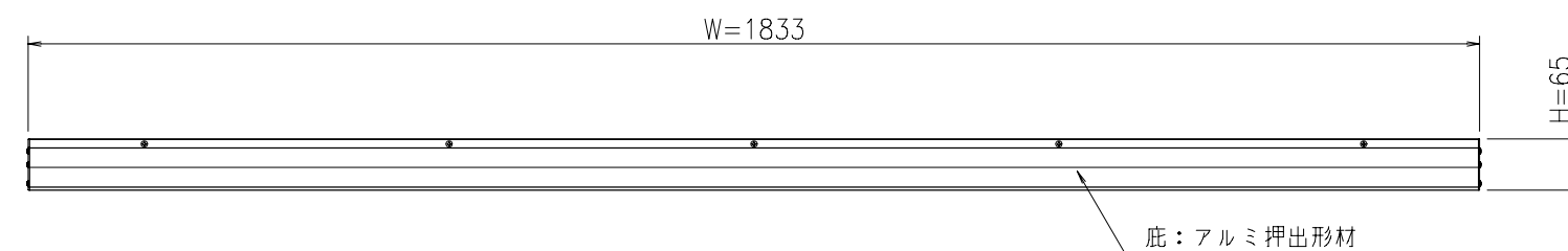
正面図
