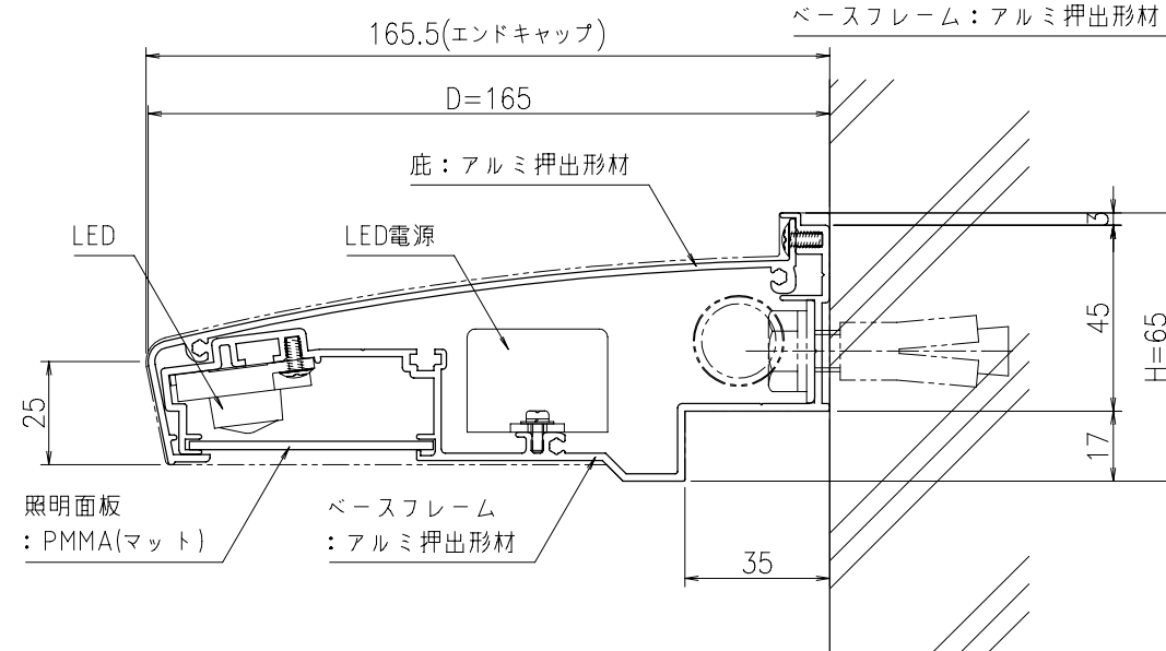
断面詳細図 (1:2)
