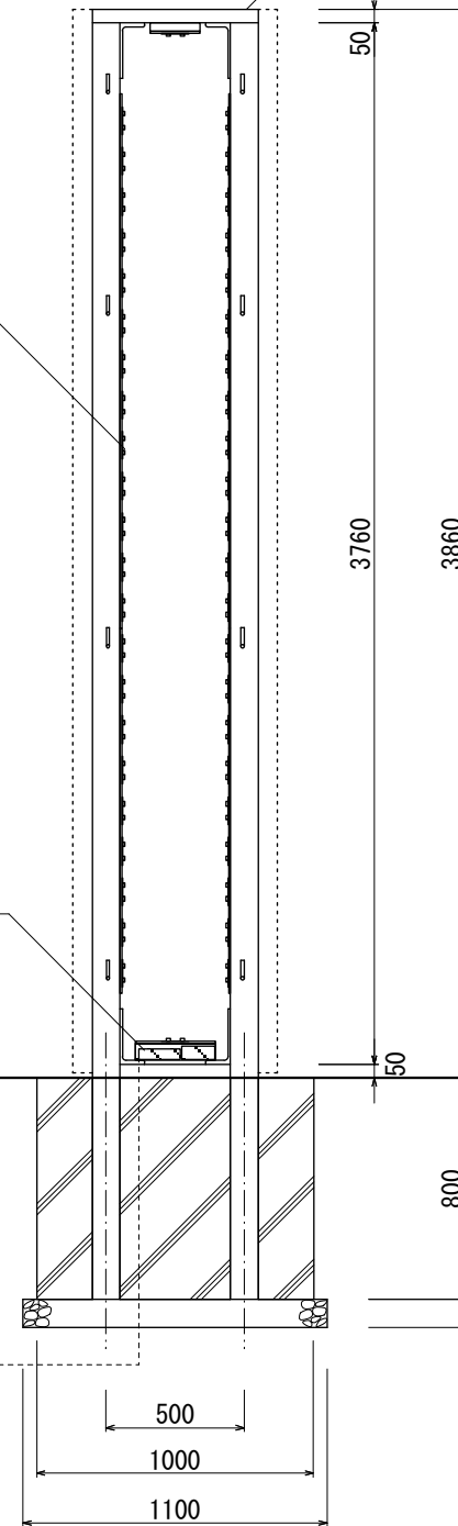
【鉄骨正面図 S=1:30】
