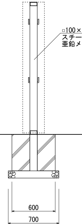
【鉄骨断面図 S=1:30】
