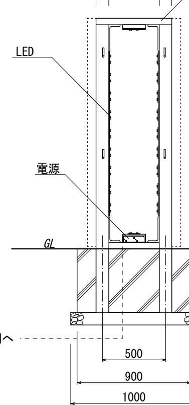
【鉄骨正面図 S=1:30】
