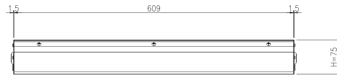
正面図
