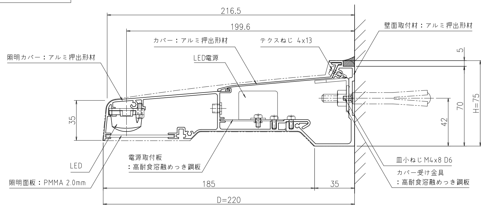
断面詳細図 (1:2)
