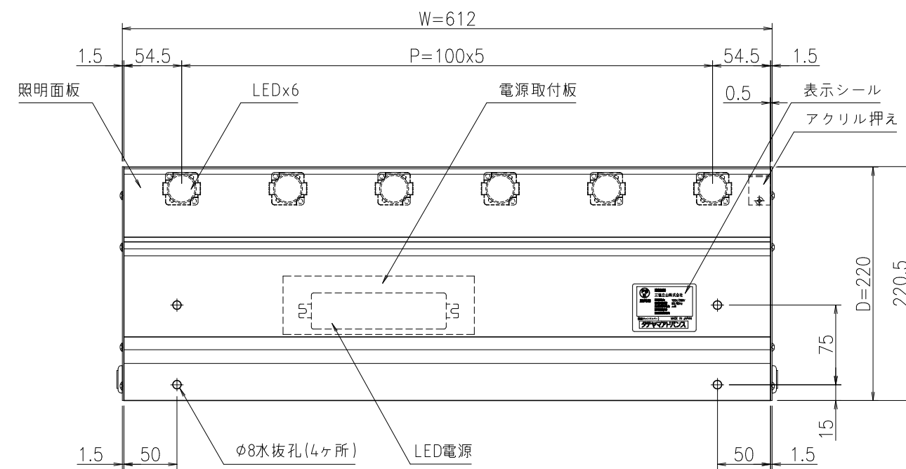
正面図
