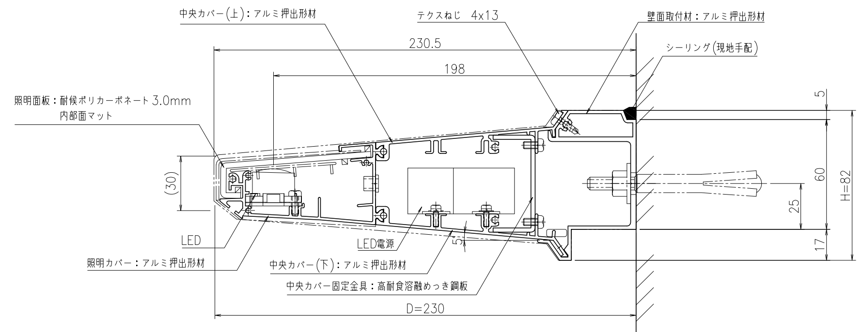
断面詳細図(1:2)
