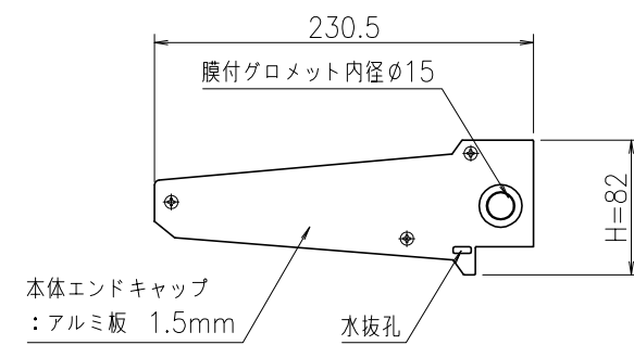
右側面図
