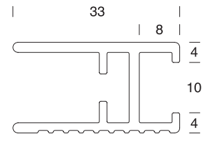
作品厚: 5mm まで UVアクリル: 2mm 見え幅: 33mm カカリ: 8mm 立ち上がり: 18mm 深さ: 10mm
