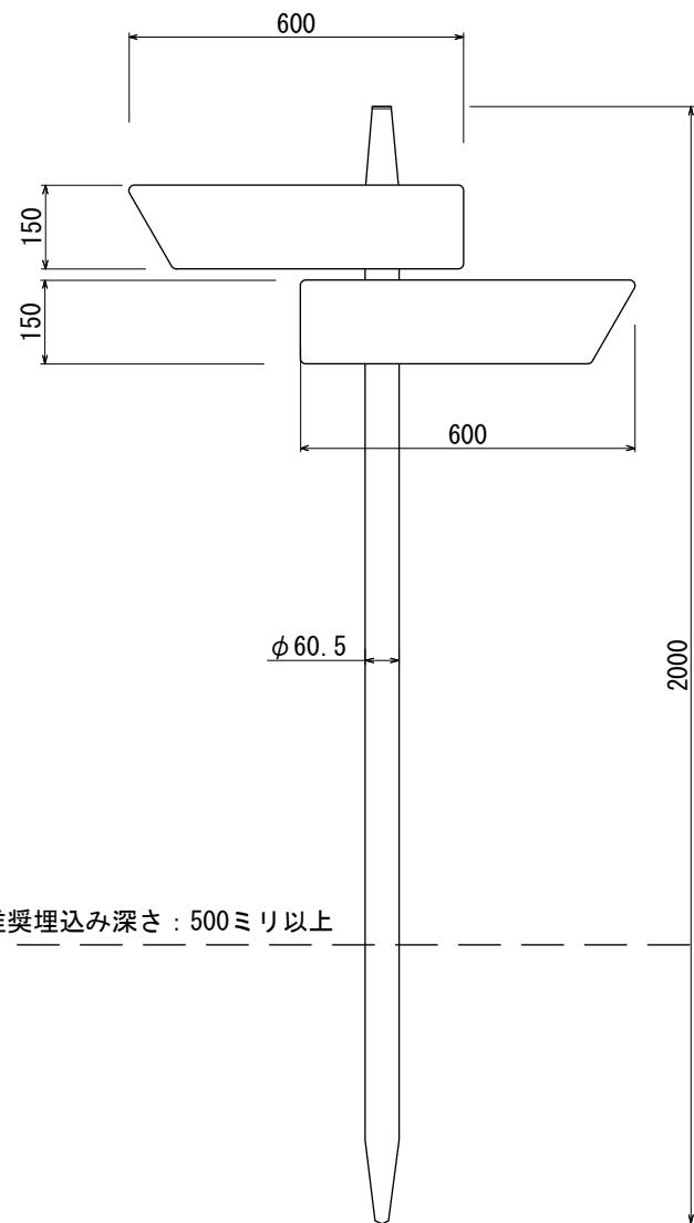
【正面図 S=1:15】
