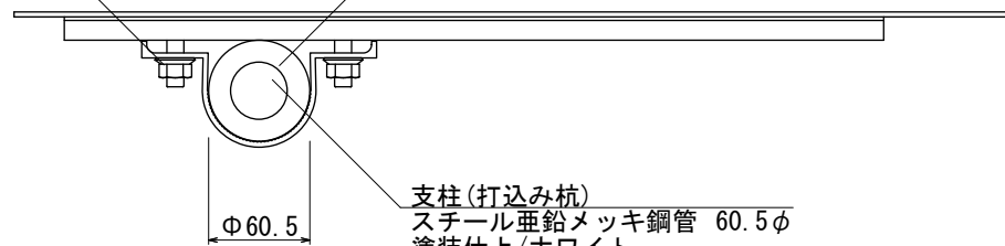
【平面図 S=1:5】
