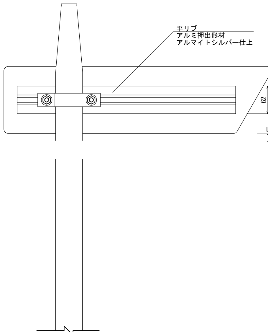
【背面図 S=1:5】
