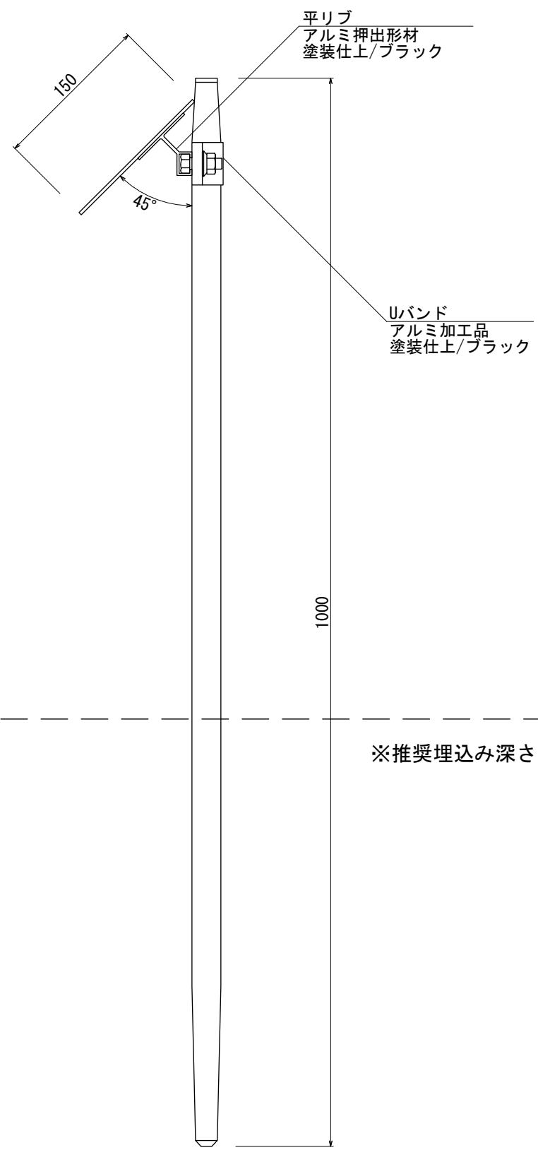
【側面図 S=1:5】
