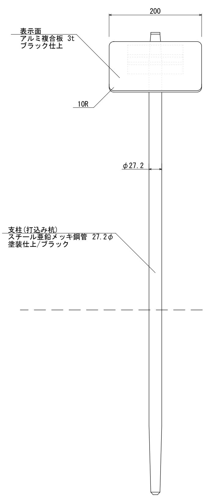
【正面図 S=1:5】
