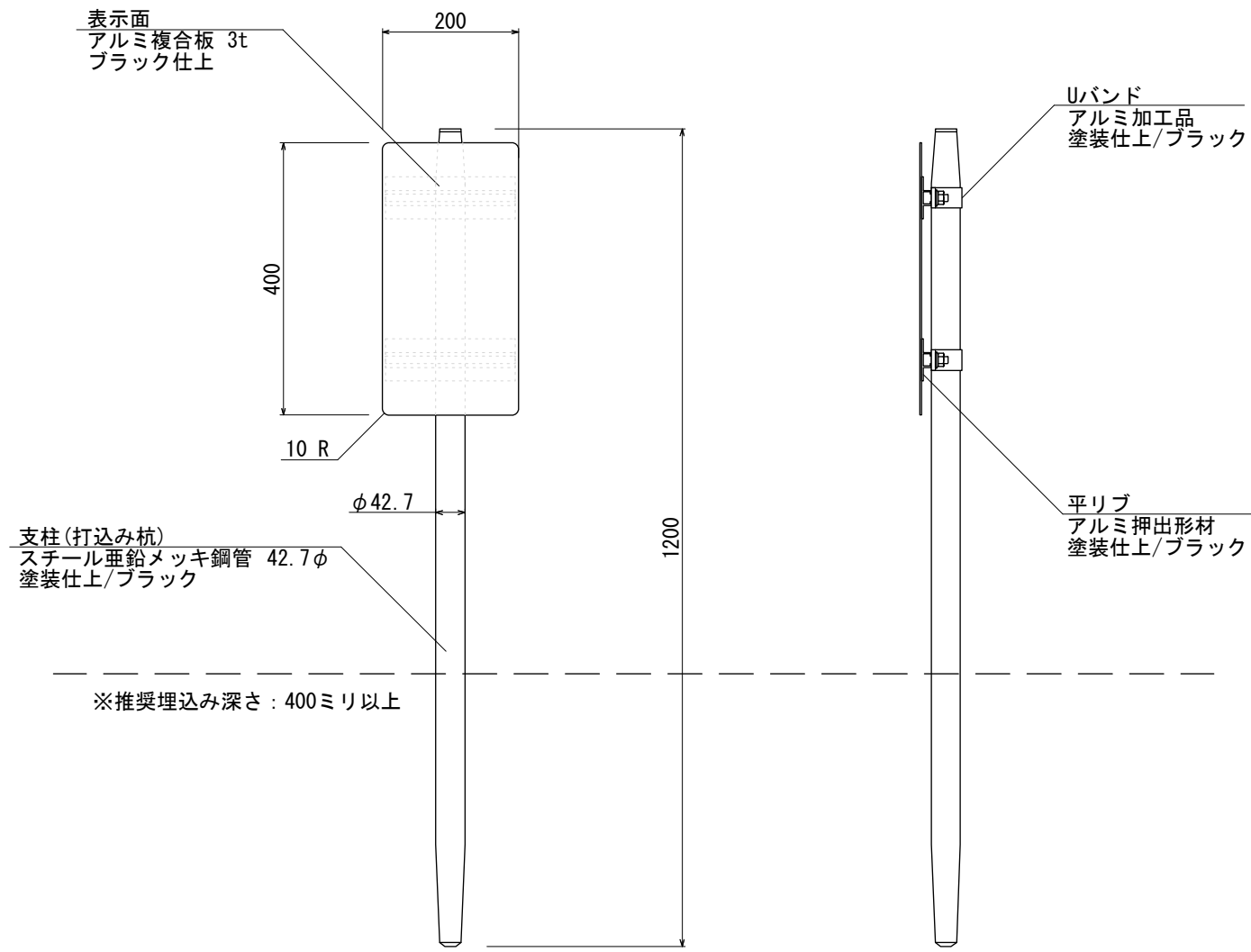
【正面図 S=1:10】
