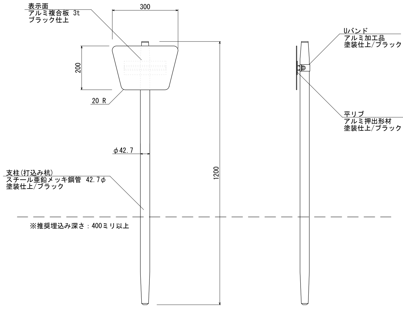
【正面図 S=1:10】
