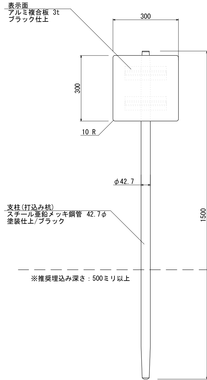
【正面図 S=1:10】
