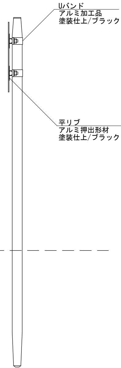
【側面図 S=1:10】
