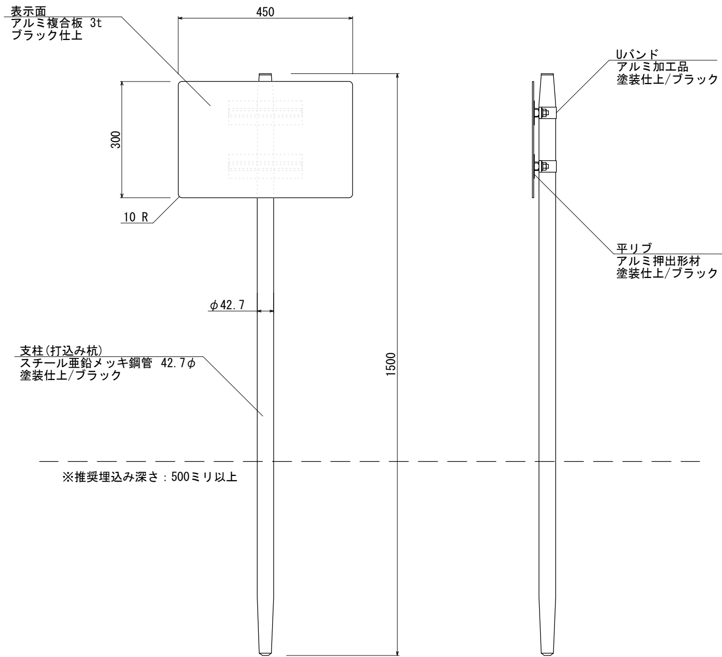
【正面図 S=1:10】
